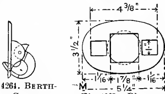
Fig. 4263. Plan.
